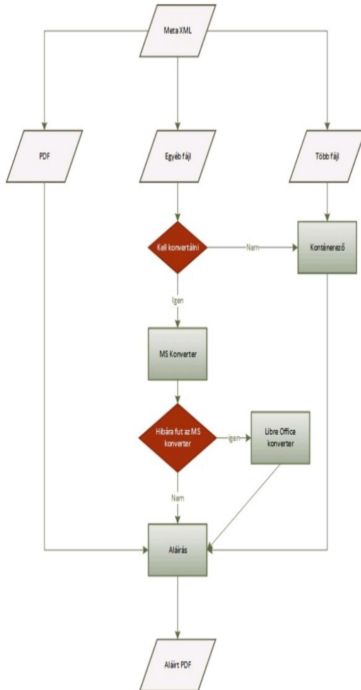
3. ábra – Az RZS Signer rendszerszintű működés
